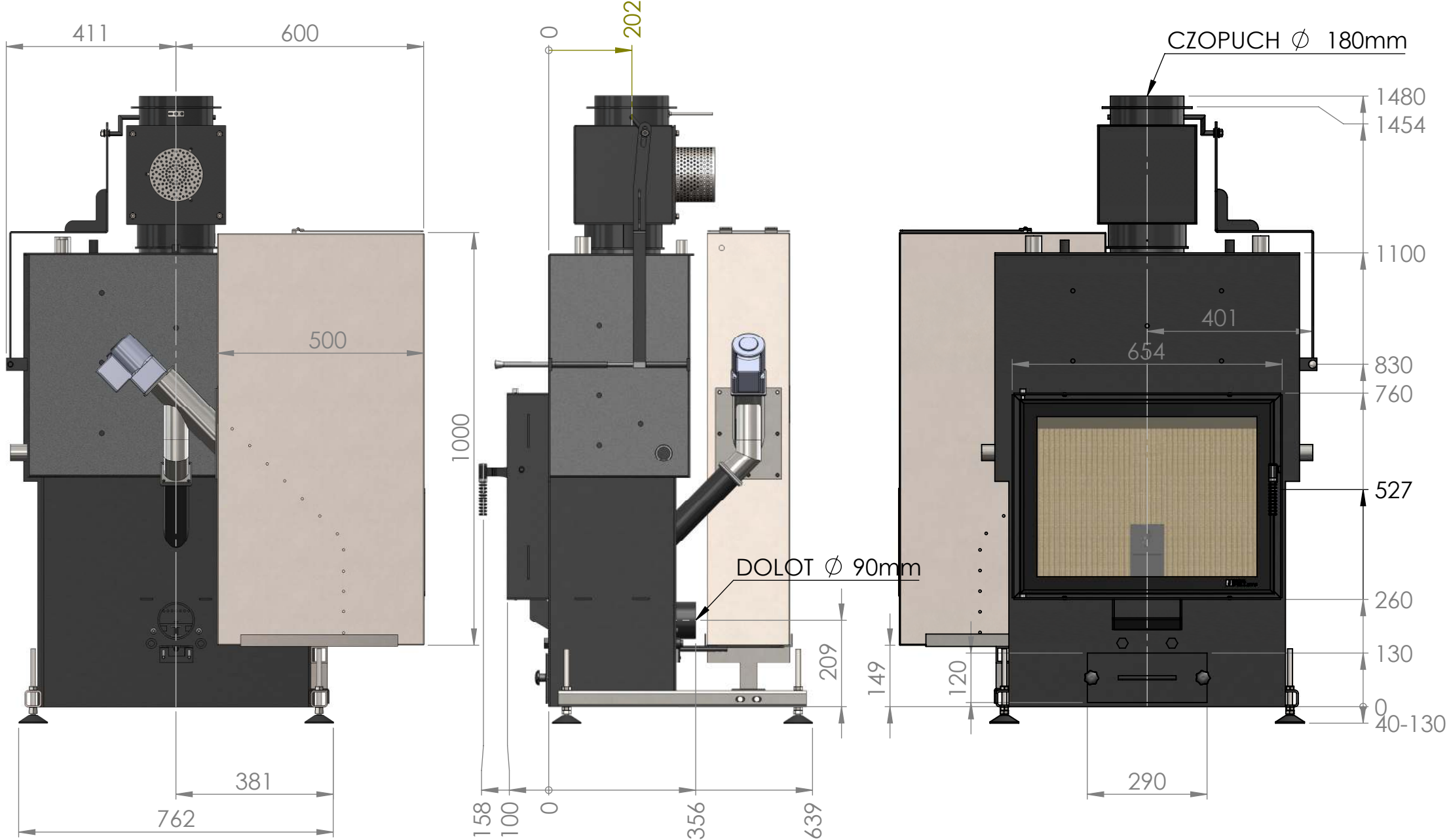
WYMIARY - LOUIS AQUA 13kW
